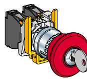
Возврат ключом (ключ № 455)
